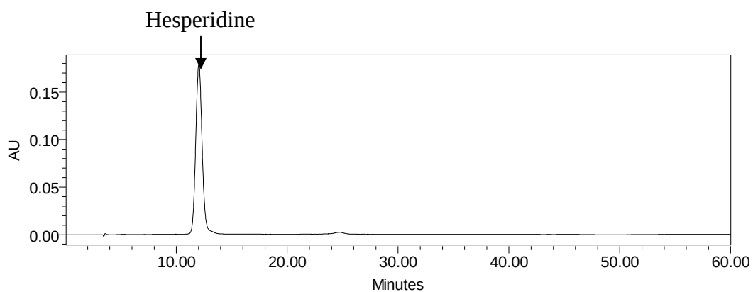
圖四、荊芥標準品 Hesperidine 之 HPLC 層析圖
