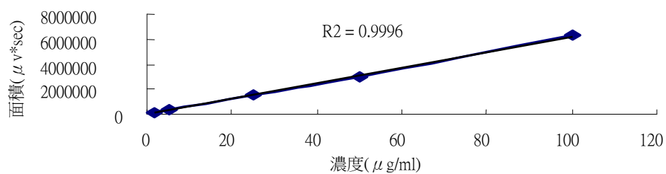
Chrysophanol 標準曲線
