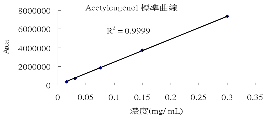
圖十七、Acetyleneugol 檢量線圖
