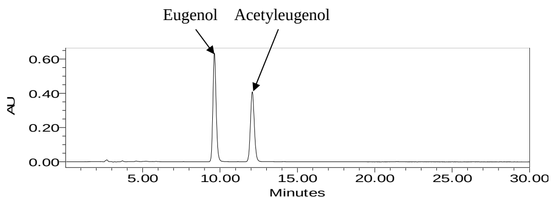
圖十四、丁香標準品 Eugenol 及 Acetyleneugenol HPLC 層析圖
